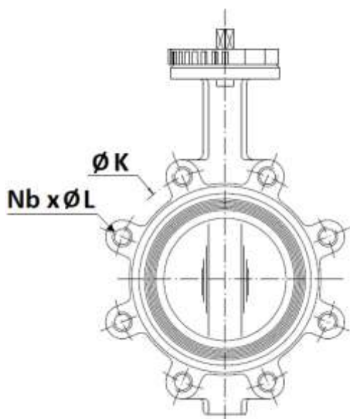
DN 32-150
